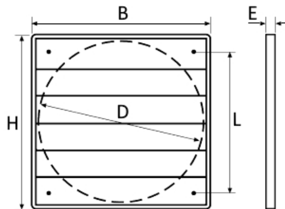
Modèle 1 : Ø250 à 500
